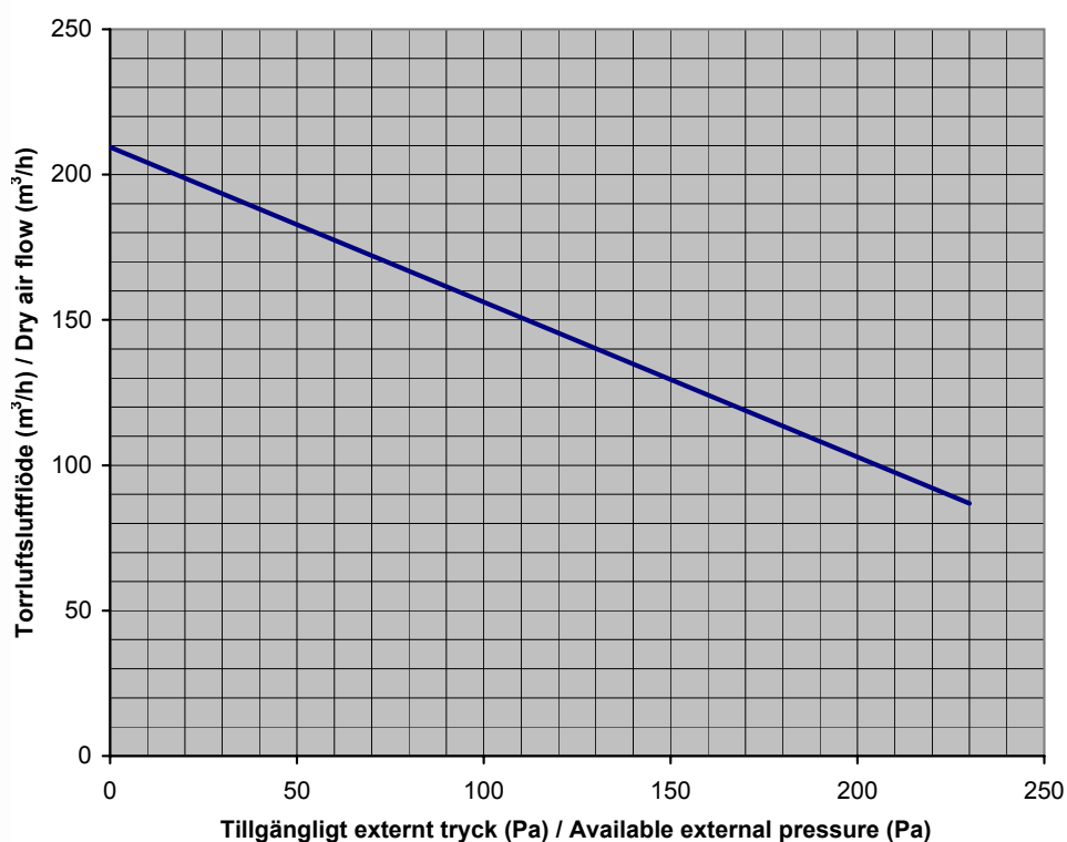
DA 210 Torrluftsflöde/Tillgängligt tryck / DT 210 Dry air flow/Available pressure
