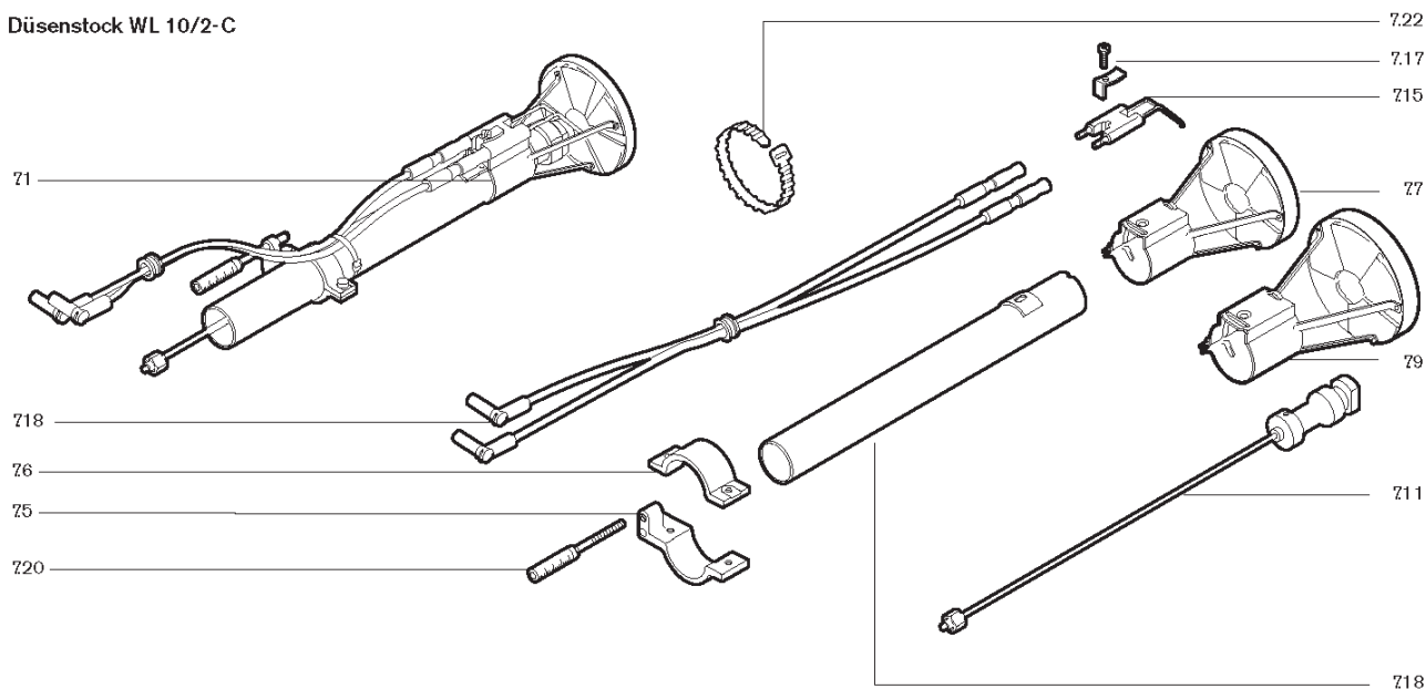
Düsenstock WL 10/2-C
