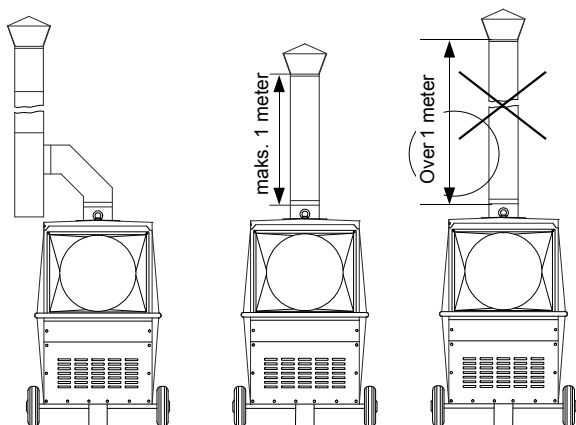
Eksempel 1 Drift med forlenget avgassrør. Kondensfelle påkrevd
