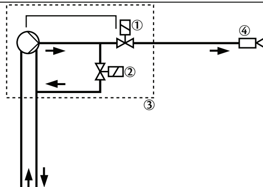
Funksjonsskjema WL 20/1-C, utf. Z
